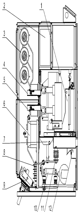
Rys. 2 Przekrój pola rozdzielnicy RDGm-12
